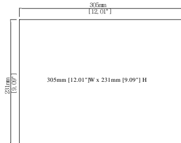
Cutout Dimensions
